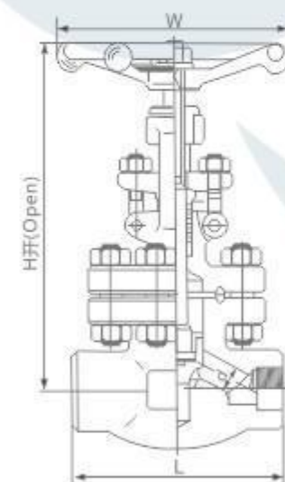
焊接阀盖示意图 Welded bonnet
